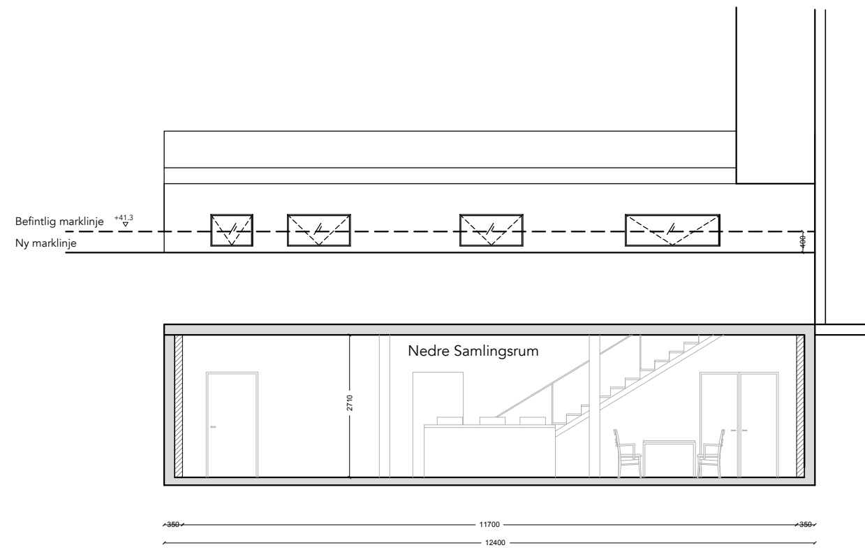
Sektion D-D
